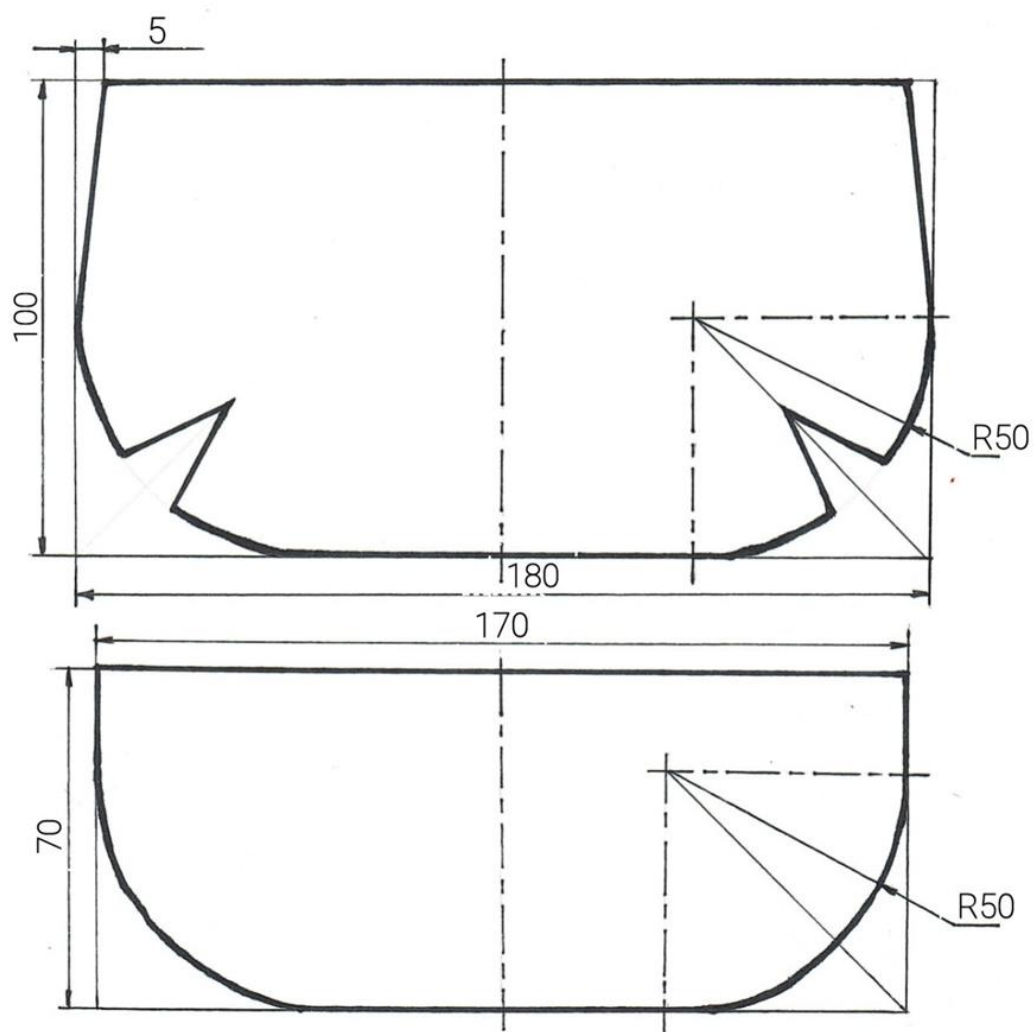
Рисунок 2. Эскиз деталей
