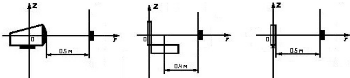
Рис. Расположение измерительной антенны относительно экранов дисплеев ВДТ, ЭВМ или ПЭВМ.
